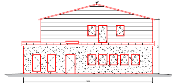
Ansicht Nord
