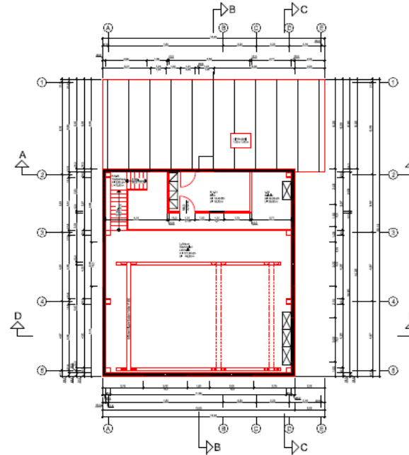
Grundriss Obergeschoss
