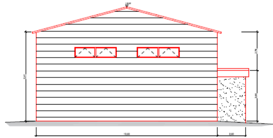
Ansicht Süd
