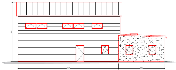
Ansicht Ost
