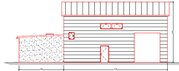
Ansicht West
